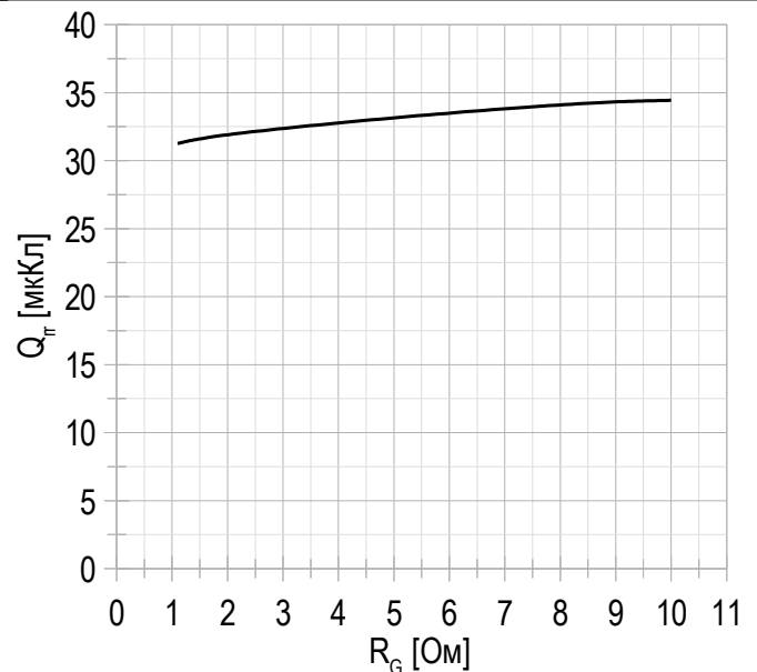
Рисунок 12 – типичная зависимость заряда обратного восстановления от сопротивления в затворе, FRD.
