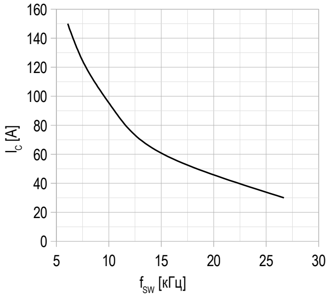
Рисунок 17 – типичная зависимость тока коллектора от частоты.
